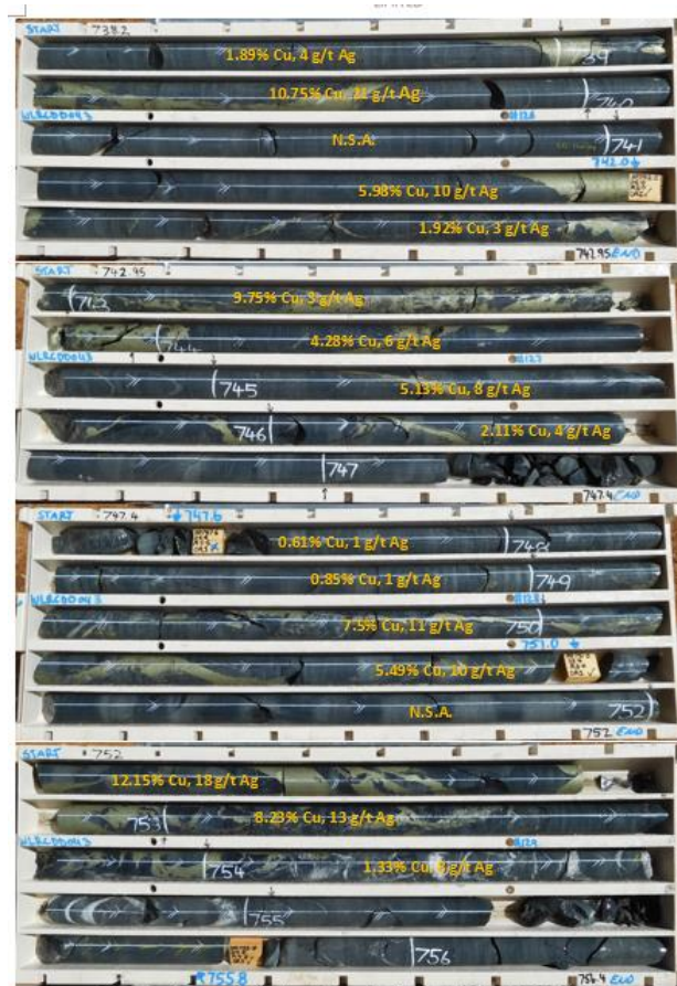
着鉱部コア写真: WLRCD043 孔 掘進長 738.00–755.00m(17m 間) 銅 4.59%、銀 8g/t、金 0.01g/t
